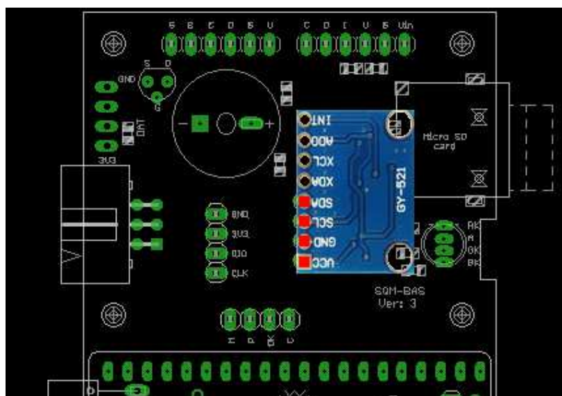
Uložení 2: Modul s 8 vývody (otáčení kolem osy X), připájený přes kolíkové lišty k SGM-BAS ver.3, čipem dolů.
