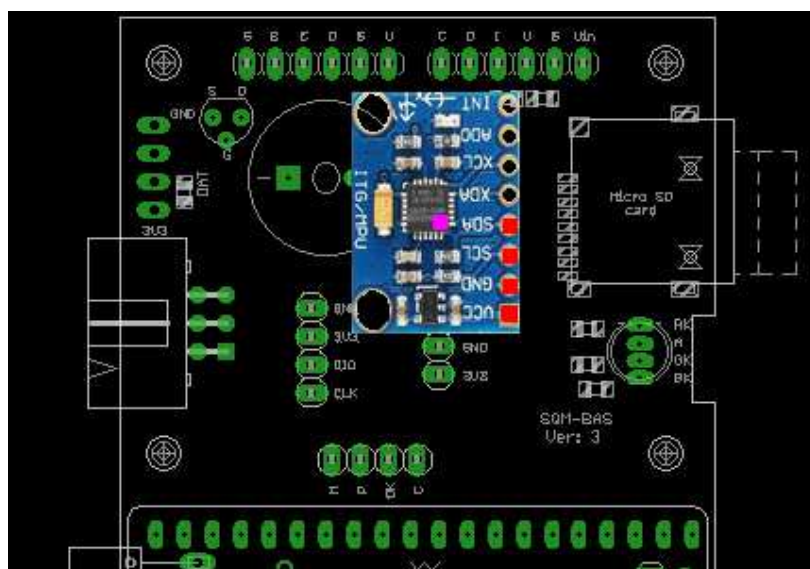
Uložení 1: Modul s 8 vývody (otáčení kolem osy X), přilepený na pískáku, čipem vzhůru. Propojení na desku SGM-BAS provedeno dráty.
